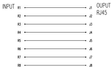
连线关系
