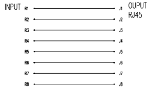
连线关系
