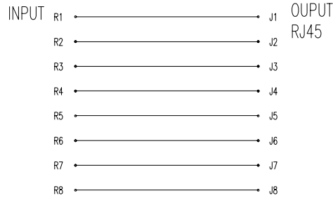
连线规则
